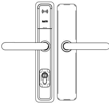
Ex7P0RO/SH (beidseitig Drücker, mechanische Notöffnung mit elektronischer Protokollierung über Halbzyylinder außen, mechanischer Zylinder nicht enthalten)
