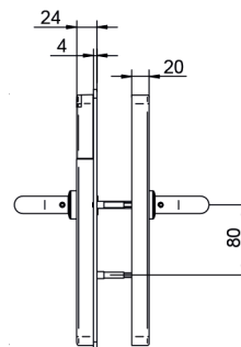
DIN Rosettenkonfiguration (RO)
