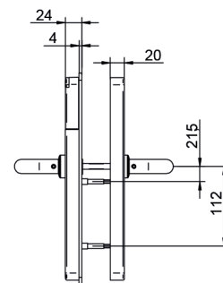
DIN Kurzschildkonfiguration (SH) 4)
