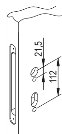
DIN-Kurzschildkonfiguration (SH) 4)
