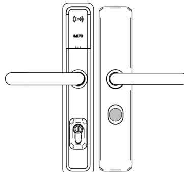
Ex7P6RO (beidseitig Drücker, mechanische Notöffnung mit elektronischer Protokollierung über Halbzyylinder außen, mechanischer Zylinder nicht enthalten, elektronische „Bitte nicht stören“-Funktion innen, ) 4)
