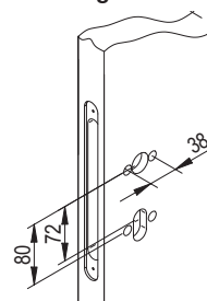
DIN-Rosettenkonfiguration (RO)
